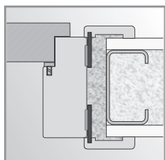
Beépítés pürhabbal gipszkarton falba
