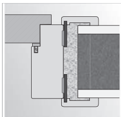
Beépítés a pürhabbal kőműves falba
