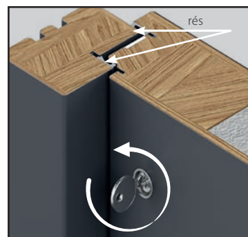
Bezárás UTÁN ~ 3 mm
