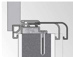
falvastagság beállítási tartomány
