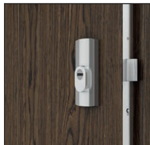
négy pontos szalagzár két cylinderbetéhez – KVARC III
