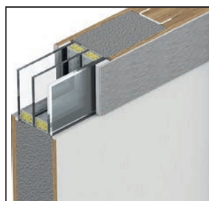
Háromrétegű meleg peremes üvegezással – P4 betörésvédelmi osztály, rozsdamentes acél kerettel
