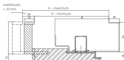
PROJECT Prémium tok metszet
