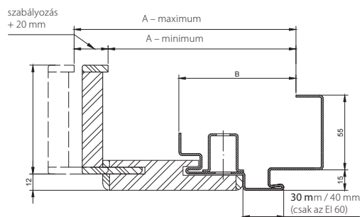
PROJECT tok metszet
