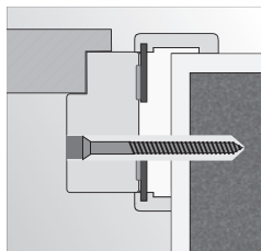
Beépítés pürhabbal és dűbellel kőműves falba
