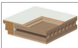
Porta többrétegű szerkezet (42 dB)
